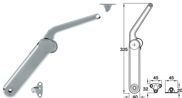
Wooden lid flap
